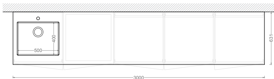
PIANTA
