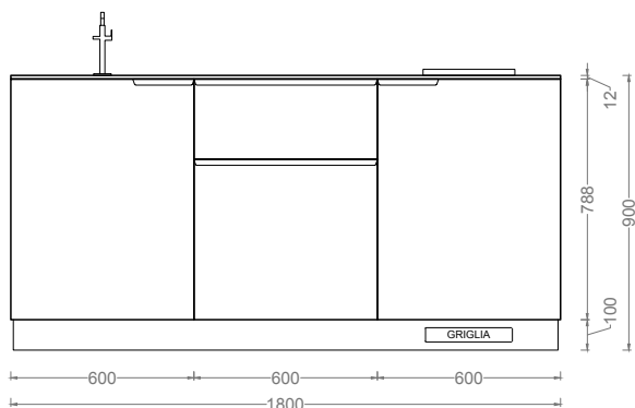
PROSPETTO FRONTALE
