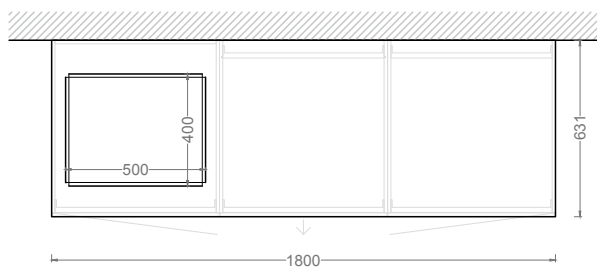
PIANTA
