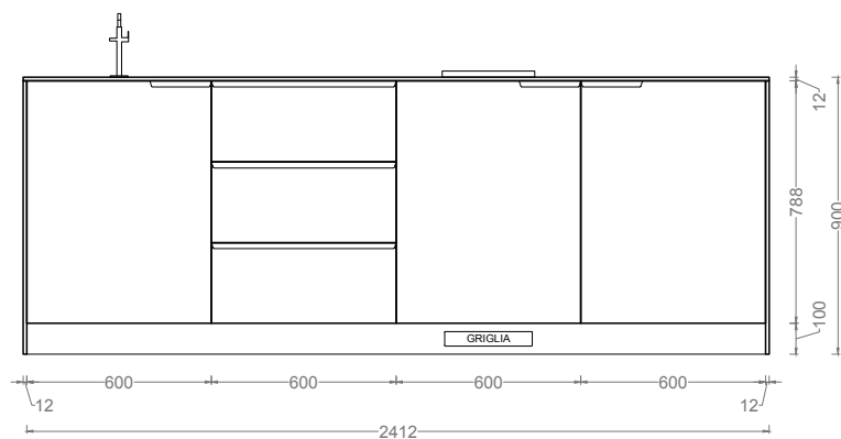
PROSPETTO FRONTALE
