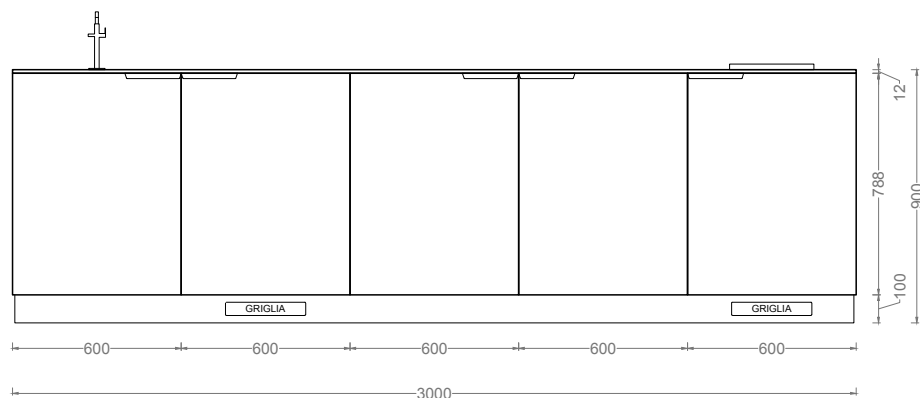
PROSPETTO FRONTALE
